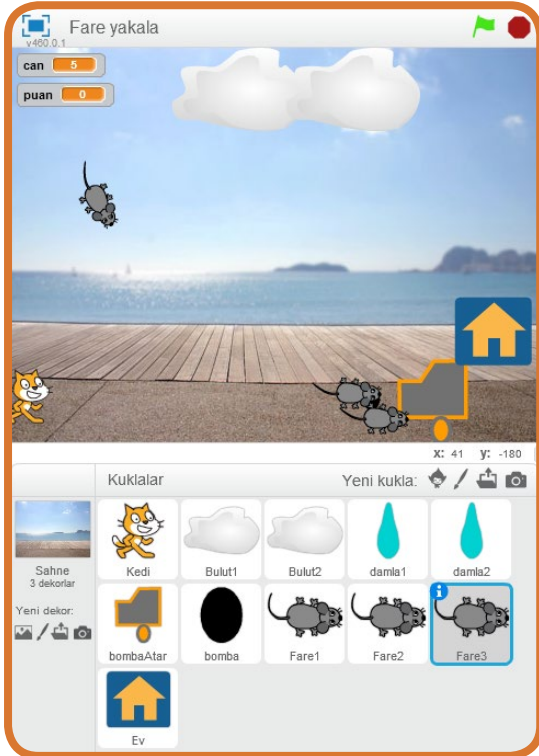
Şekil 100: Fare yakalama oyunu sahne tasarımı
